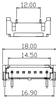
LCDMR-7P2TW
