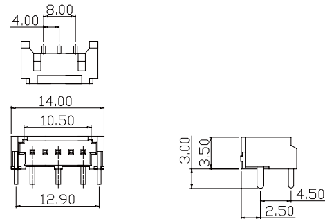
LCDMR-5P3TW
