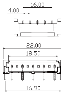
LCDMR-9P5TW
