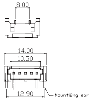
LCDMR-5P2TW
